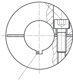
Klemnav
